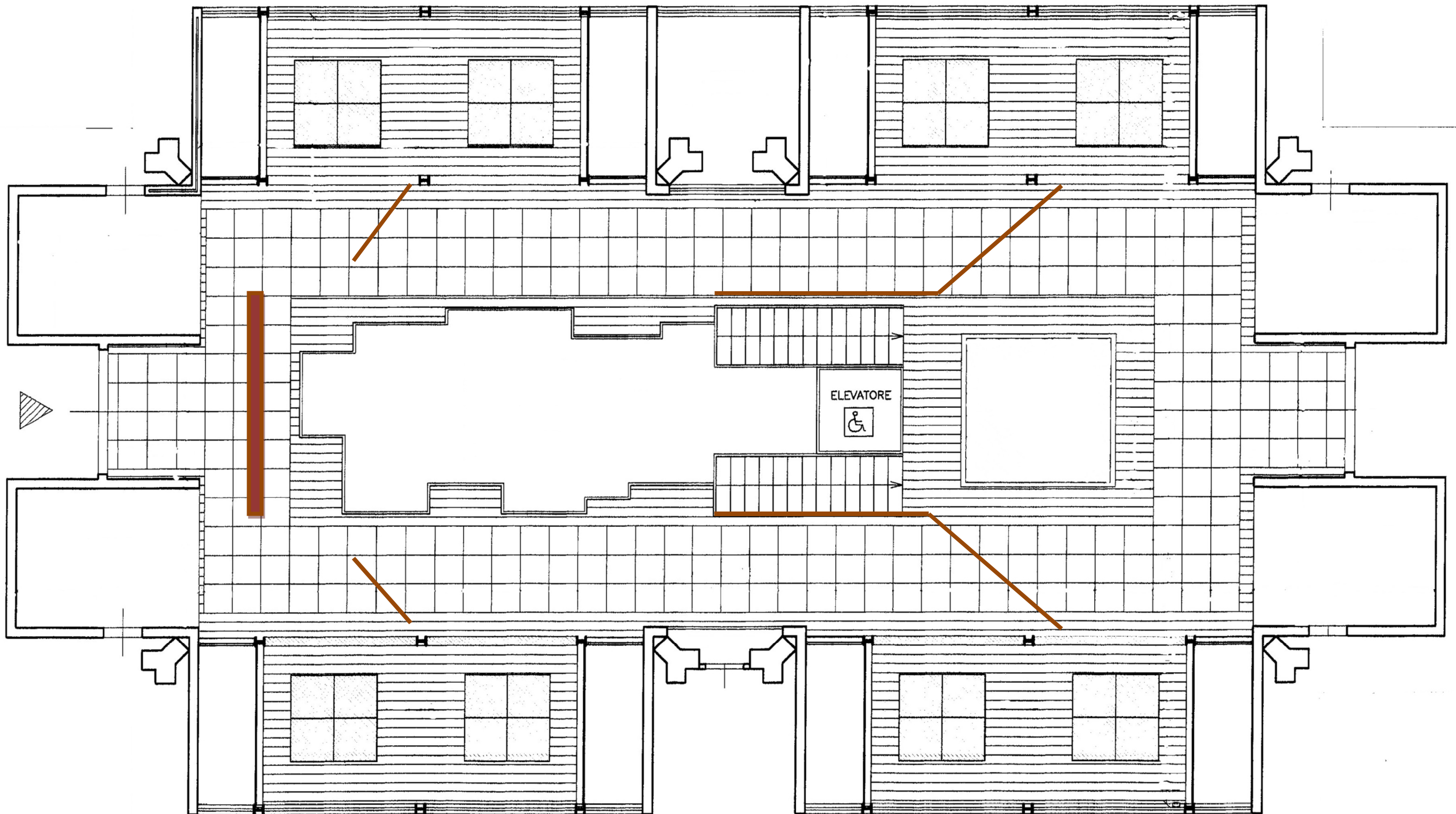
Tavola 3 - Schema delle pannellature principali di progetto (in colore)
